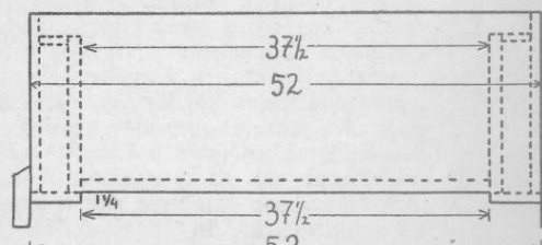
Broedkamer van voren De breedte van de vlieggatschuif, welke met 37 cm is aangegeven, kan ook tot bijv. 32 cm worden teruggebracht.
