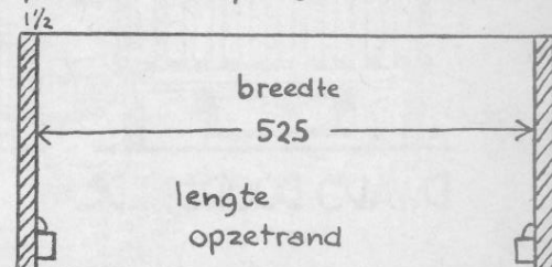
Bodemplank van terzijde (Breedte bodem 52.5)
