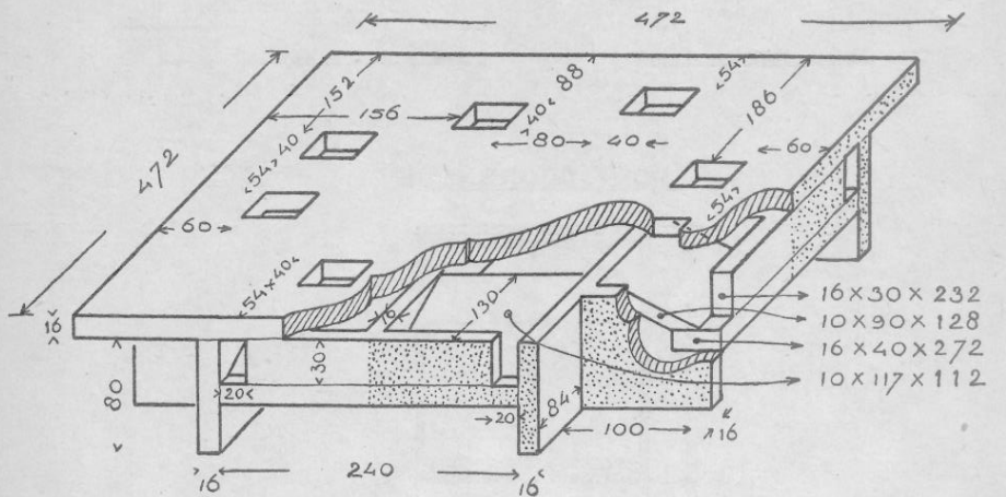
BODEMPLANK voor 8 BEVR. KASTJES
