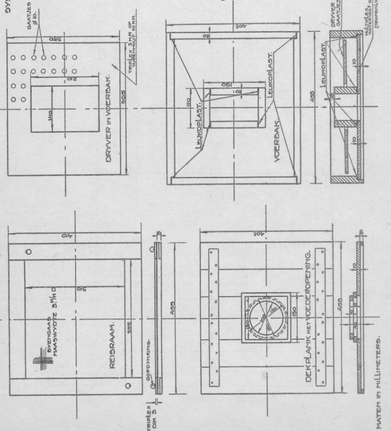
ONDERDELEN VOOR BYENKAST.
